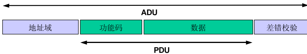
图 2：通用 MODBUS 帧
