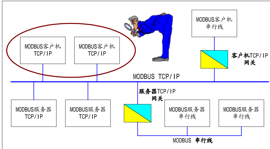
图 10: MODBUS 客户端
