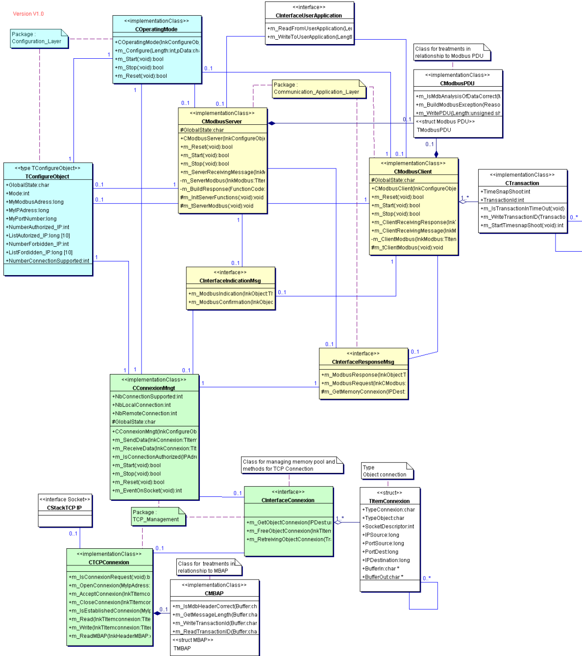
图 22: 类的示意图
