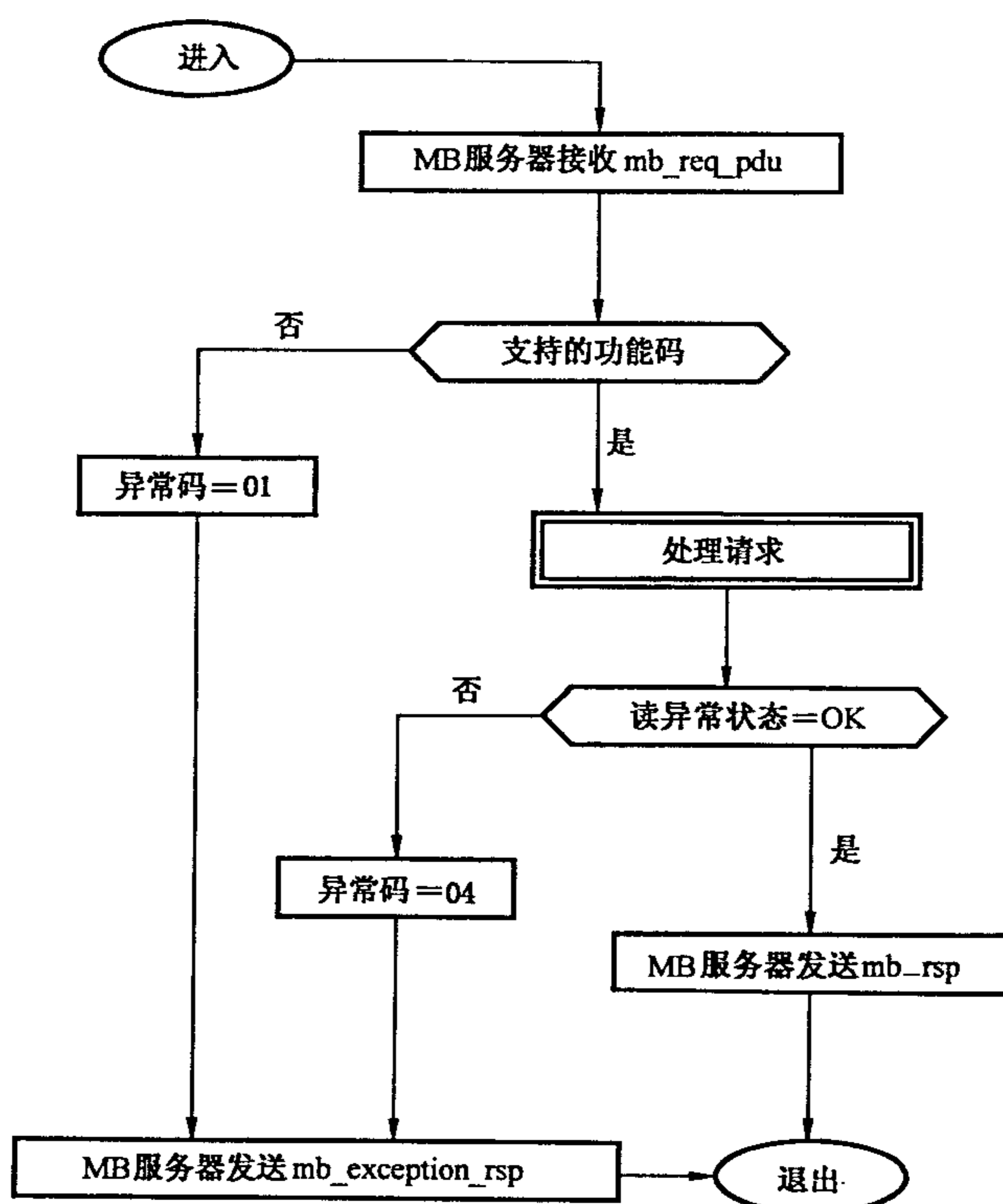
图 17 读异常状态的状态图
