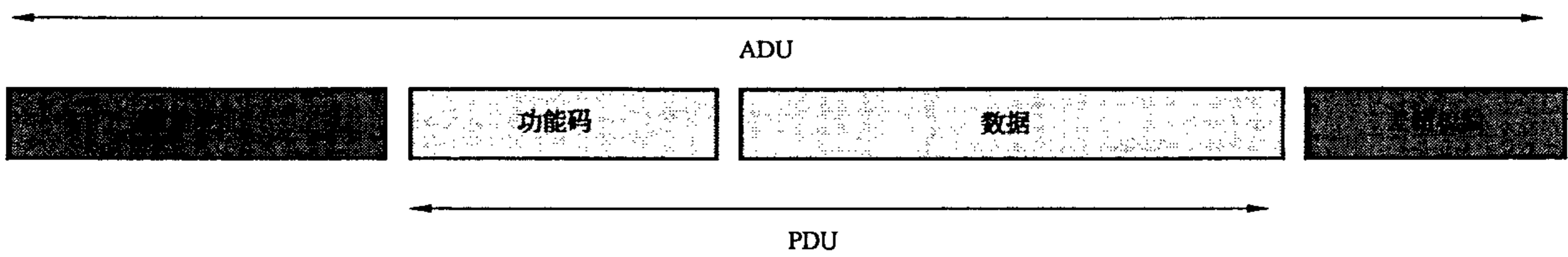
图 3 通用 Modbus 帧
