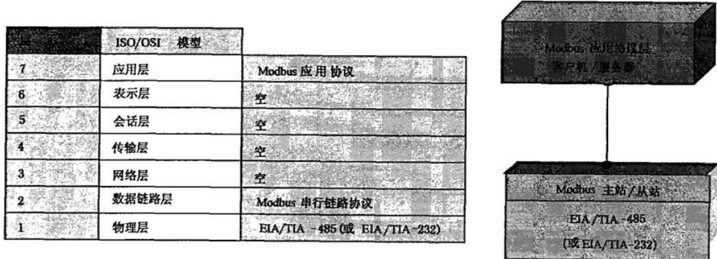
图 2 Modbus 协议和 ISO/OSI 模型
