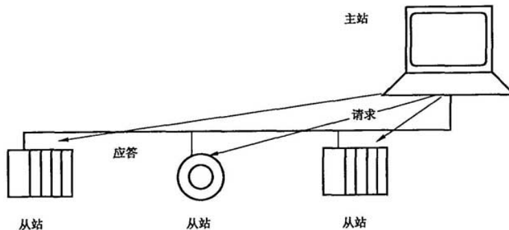
图 4 广播模式
