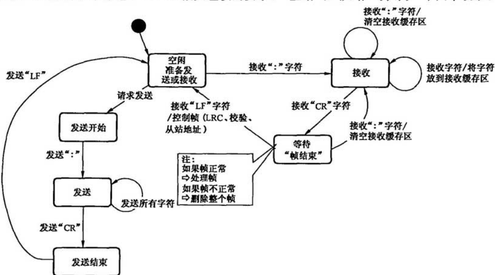
图 20 ASCII 传输模式的状态图
