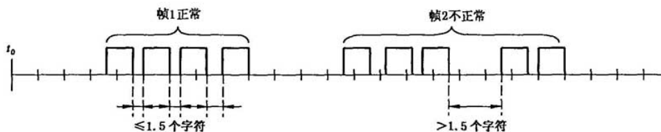
图 15 Modbus 帧内间隔
