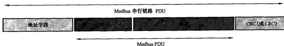
图 6 串行链路上的 Modbus 帧
