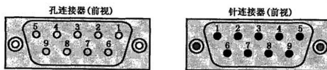
图 27 9 针 D-型连接器
