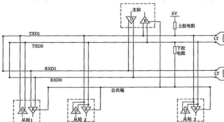
图 24 将 4 线接线系统转换为 2 线接线系统
