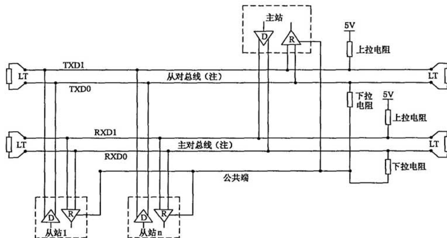
图 23 通用的 4 线拓扑结构
