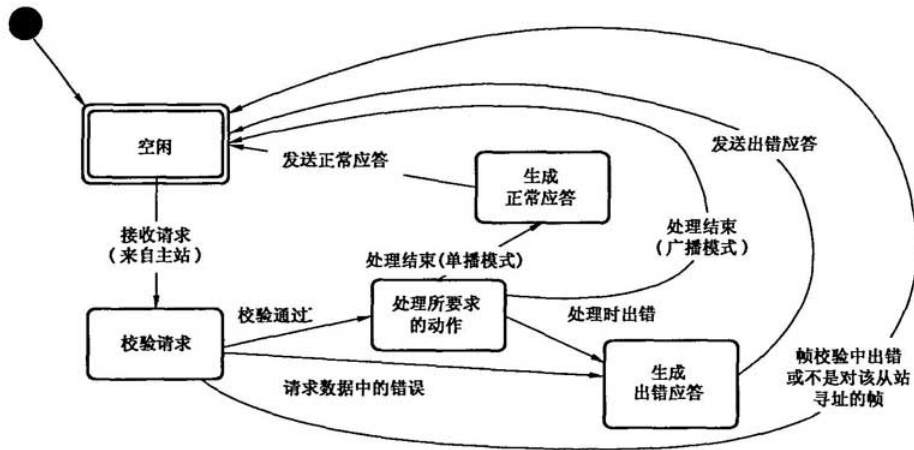
图 9 从站状态图
