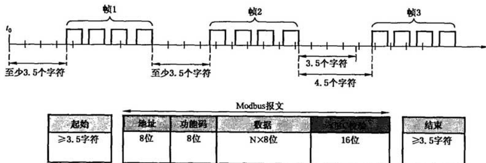
图 14 RTU 报文帧
