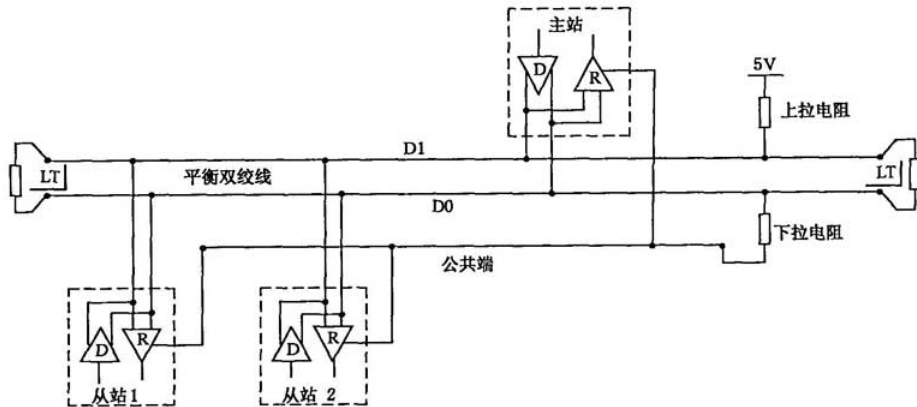
图 22 通用的 2 线拓扑结构
