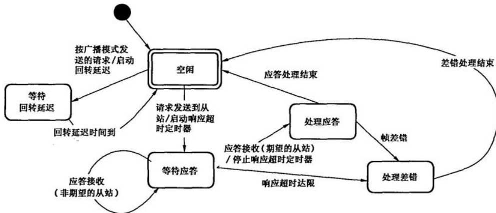
图 8 主站状态图
