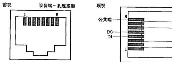
图 26 2 线 Modbus 中使用的 RJ45 连接器(要求的插脚引线)
