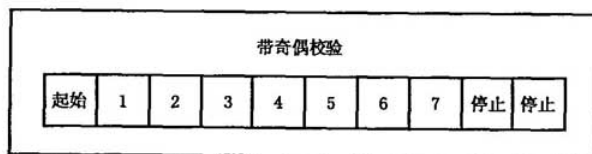
图 17 ASCII 模式中的位序列
