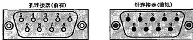
图 29 9 针 D-型连接器
