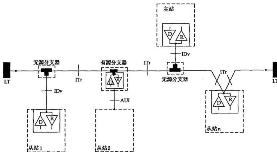
图 21 串行总线结构
