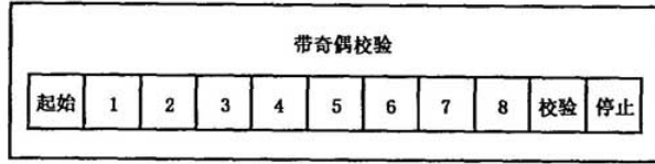
图 11 RTU 模式中的位序列
